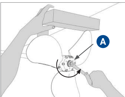
FIG. 10 | Dévisser l'écrou de serrage
