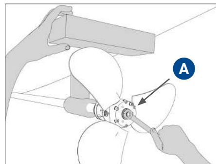
FIG. 14 | Bloquer la rotation et visser l'écrou de serrage
