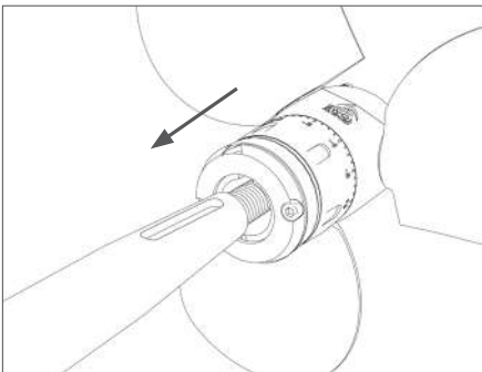
FIG. 7 | Introduction de l'hélice sur l'arbre sans clavette
